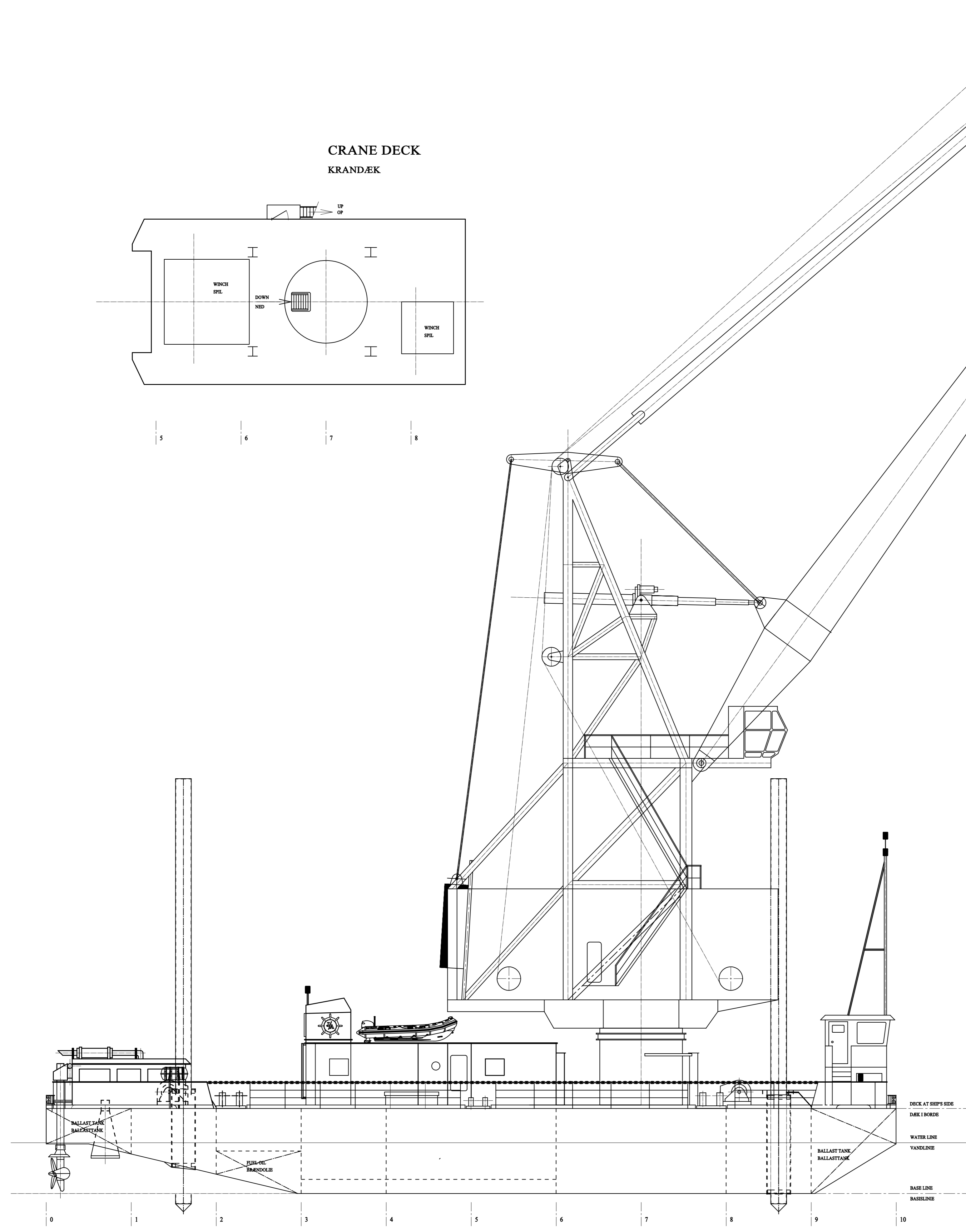
ELEVATION - SB OPSTALT - SB
